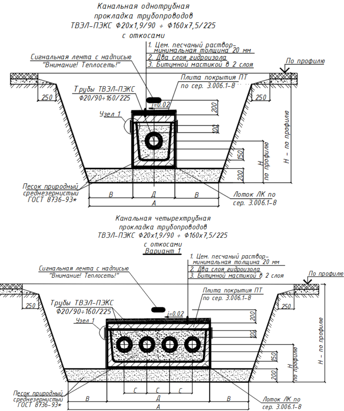
Рис. 7 Прокладка трубопроводов ТВЭЛ-ПЭКС в непроходном канале в траншее с откосами
