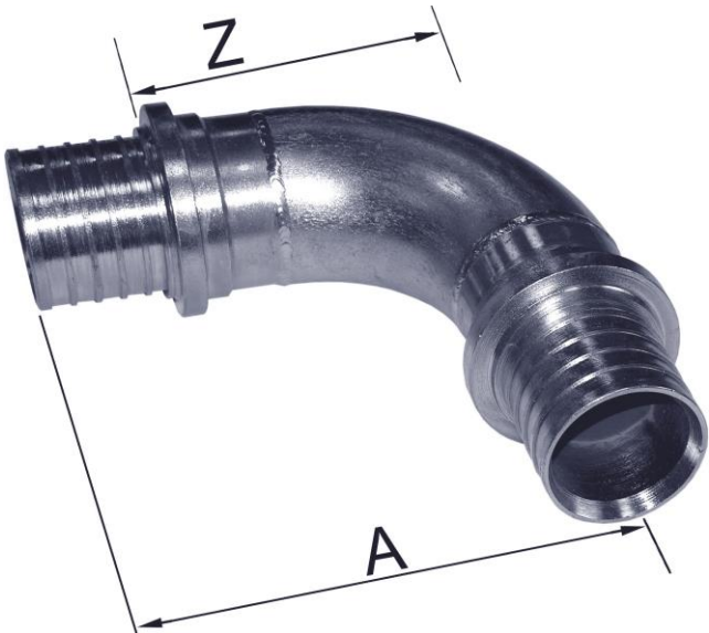
Рис.23. Угольникё
