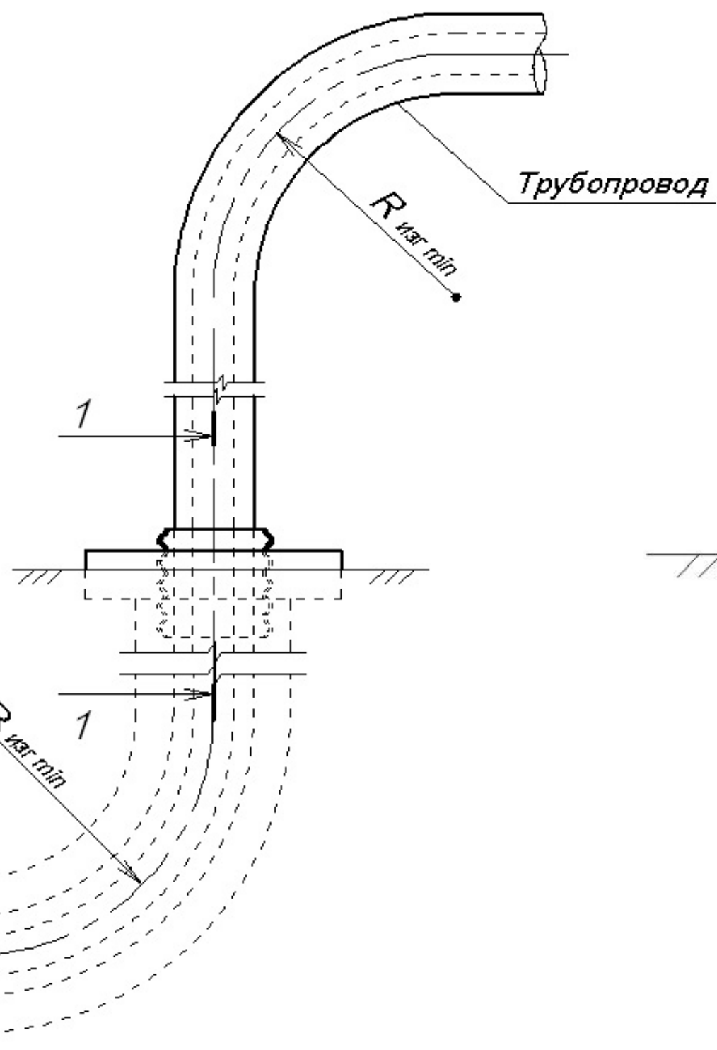
Рис. 37 Пример совмещения подземной и наземной прокладки
