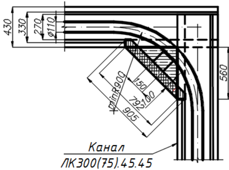
03) Закругление одностру́бной прокладки трубопроводов ТВЭЛ-ПЭКС в оболочке 180мм, 225мм
