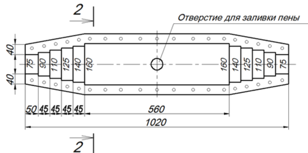
Рис. 28 Кожух для изоляции линейного стыка (для диаметров оболочек 160-225 мм)
