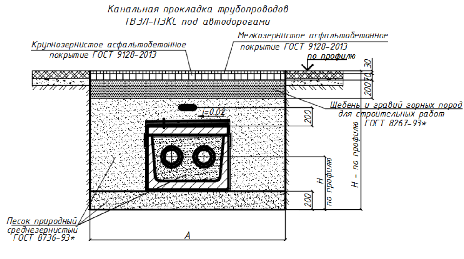
Рис. 6 Прокладка трубопроводов ТВЭЛ-ПЭКС в непроходном канале под автодорогами и газонами
