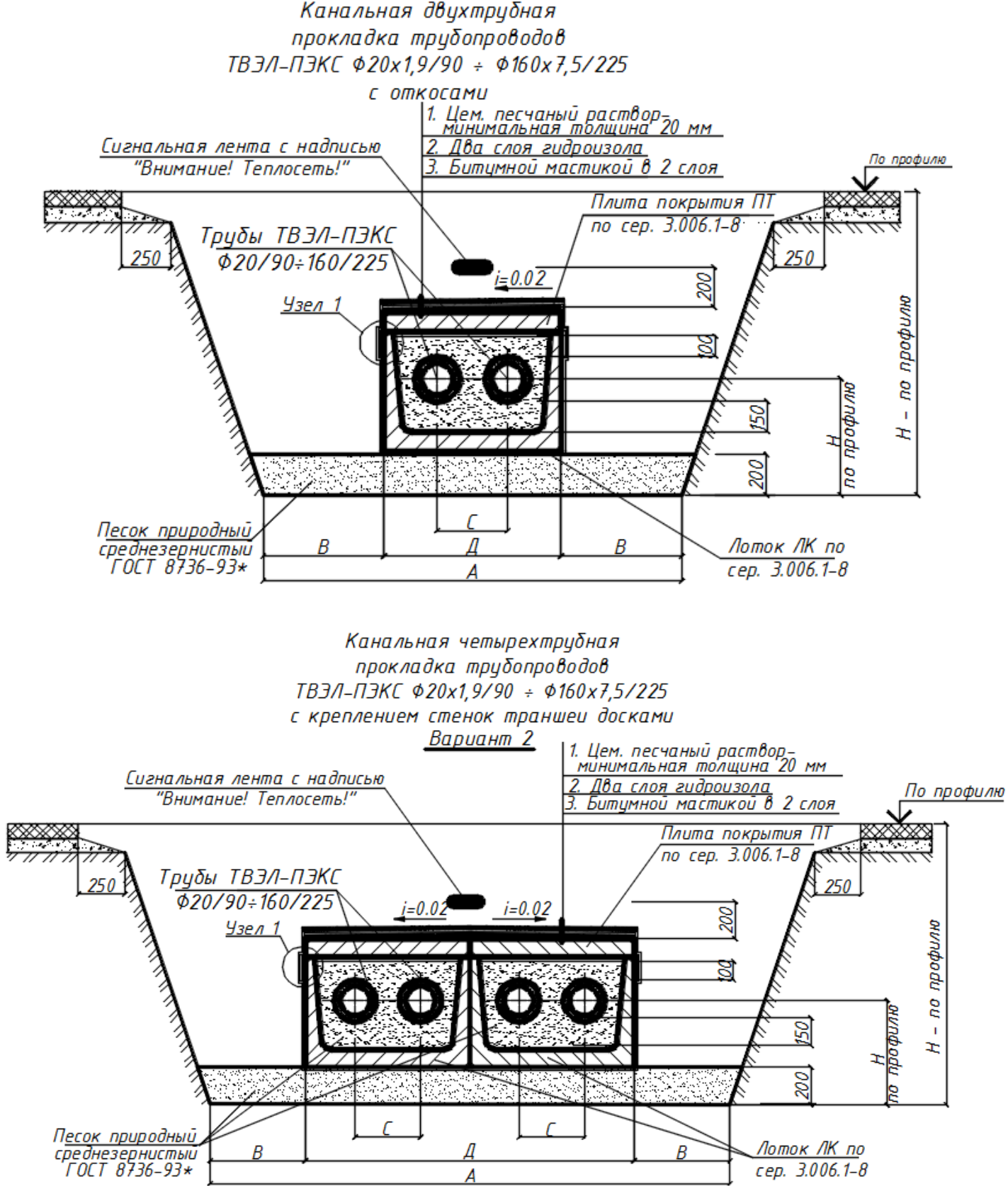
Рис. 7 Прокладка трубопроводов ТВЭЛ-ПЭКС в непроходном канале в траншее с откосами
