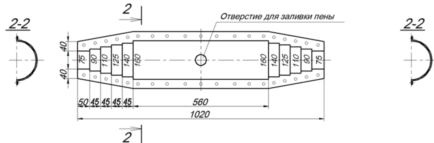
Рис. 29 Кожух для изоляции линейного стыка, универсальный (для диаметров оболочек 90-160 мм)
