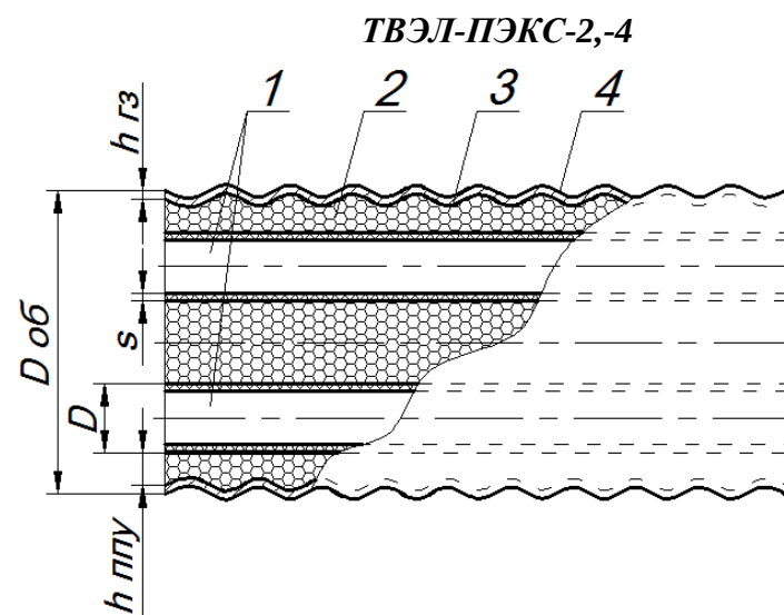
Рис. 2. Схема конструкции гибких теплоизолированных труб ТВЭЛ-ПЭКС
