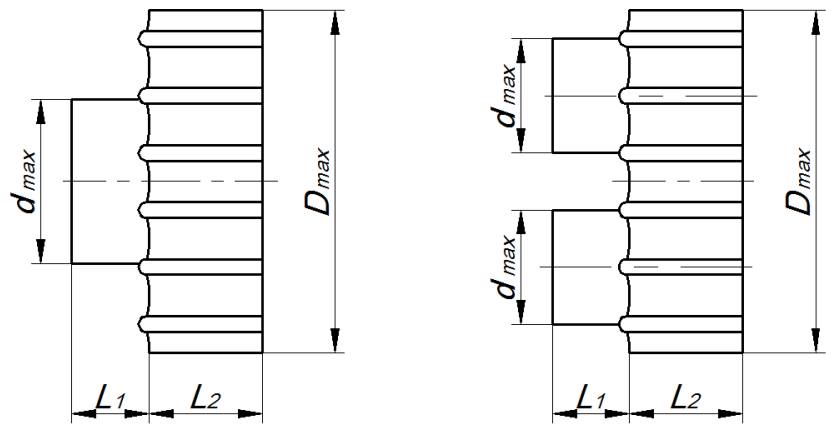
Рис. 30 Термоусаживающаяся заглушка
