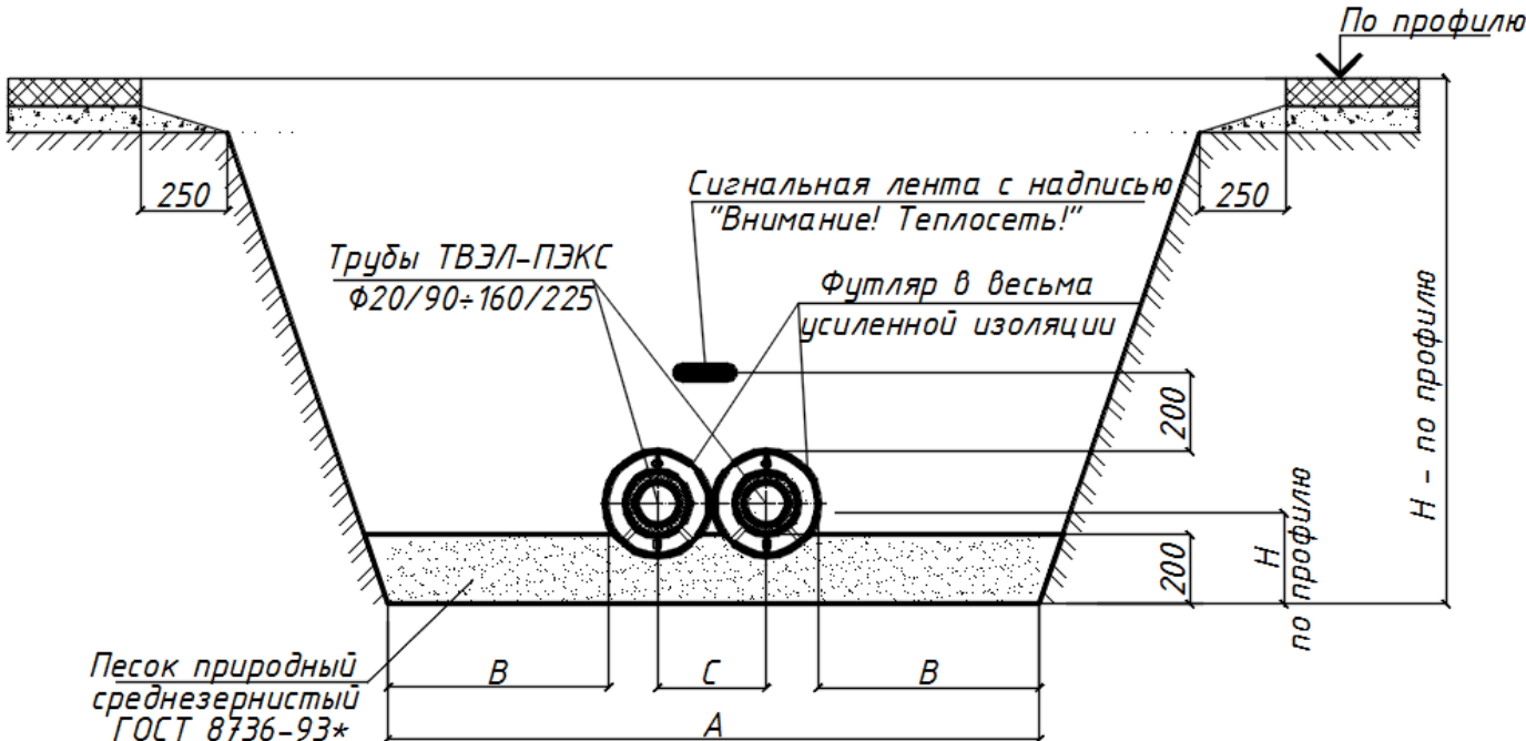
Футлярная двухтрубная прокладка трубопроводов ТВЭЛ-ПЭКС \Phi 20 \times 1,9/90 \div \Phi 160 \times 7,5/225 с откосами
